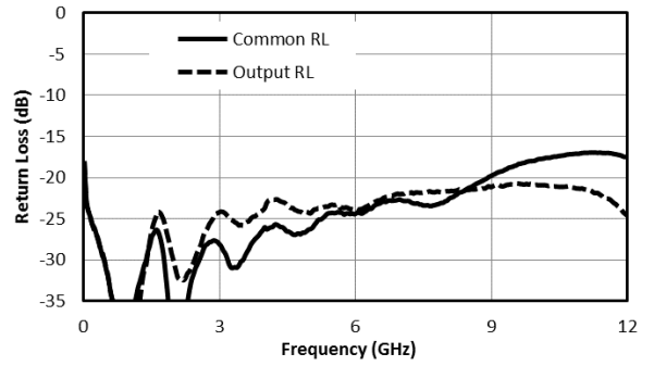
Fig. 2. Return loss
