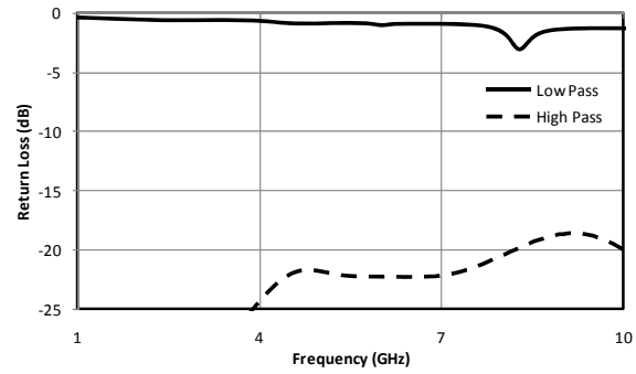
Fig. 7. Return loss.
